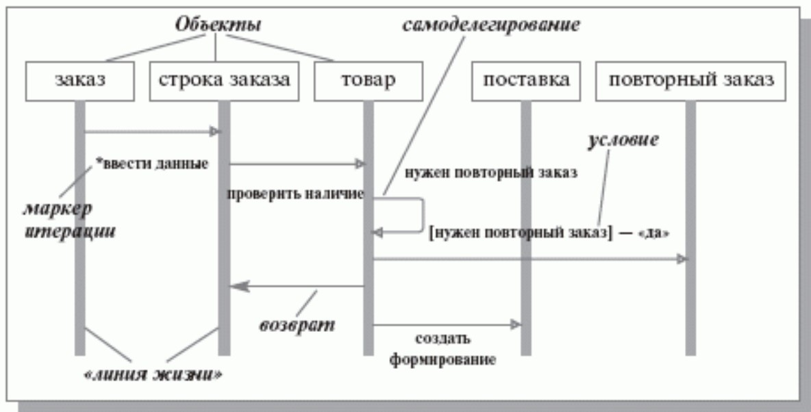
Диаграмма последовательности
