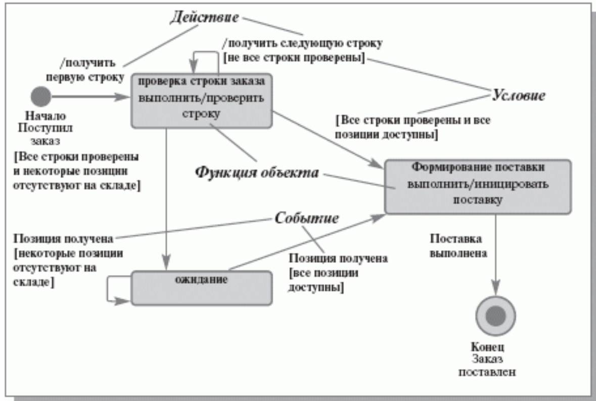
Диаграмма деятельности
