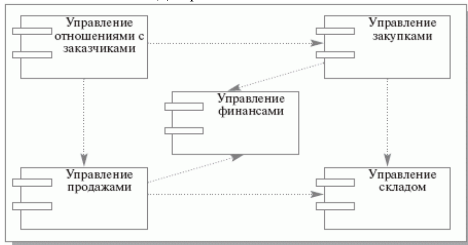
Диаграмма компонентов
